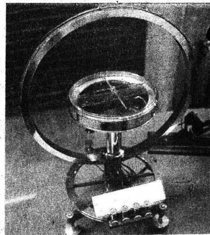
Bobina de Helmholtz.
