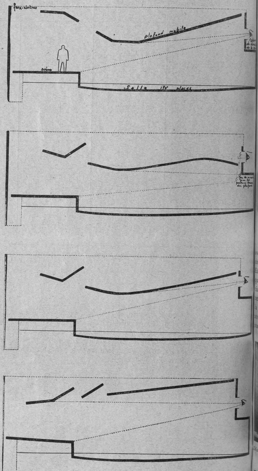
Diferentes posiciones del plafond móvil
