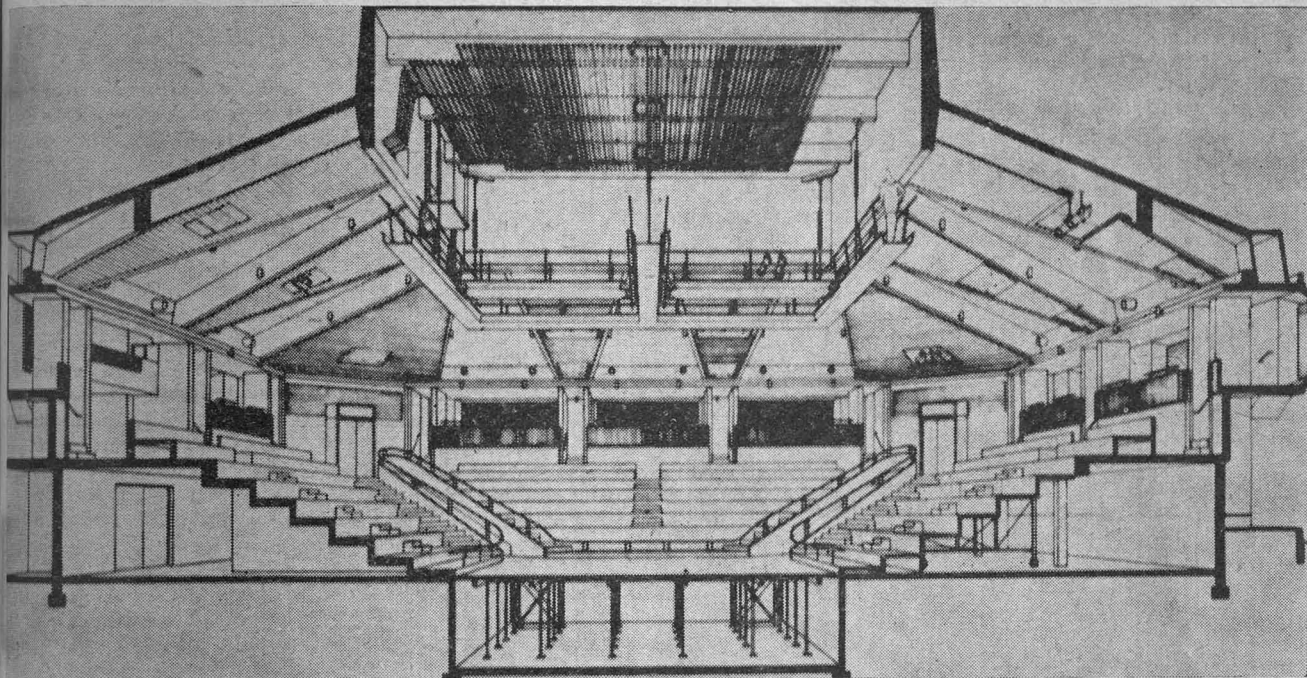
The Arena Stage, Washington D. C. (1961). Corte de la sala y del escenario. Arquitecto: Harry Weese
