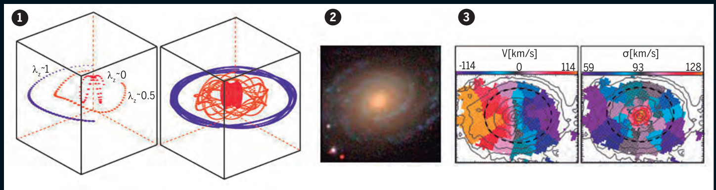
● 1) Modelo de superposición de órbitas de una galaxia, 2) observaciones hechas con el telescopio del proyecto Sloan Digital Sky Survey (SDSS) y 3) mapas de velocidad media y dispersión efectuadas con CALIFA.
